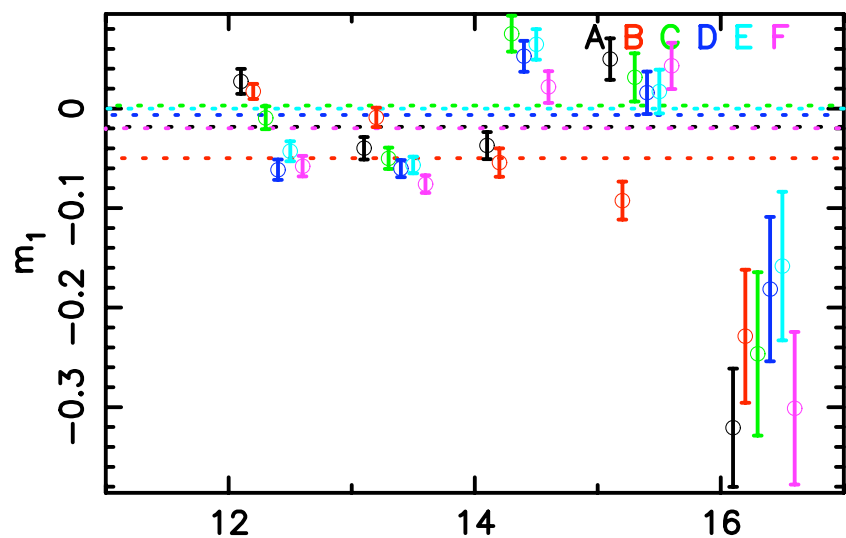
Magnitude
