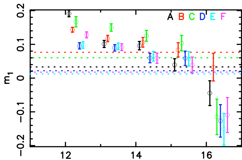
Magnitude
