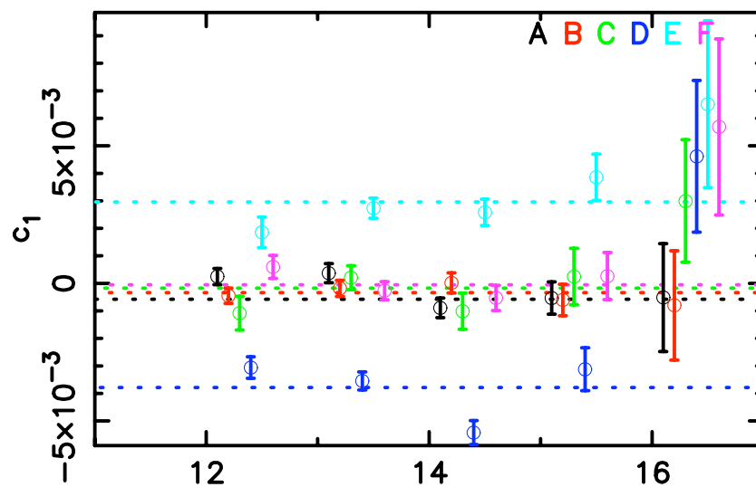
Magnitude
