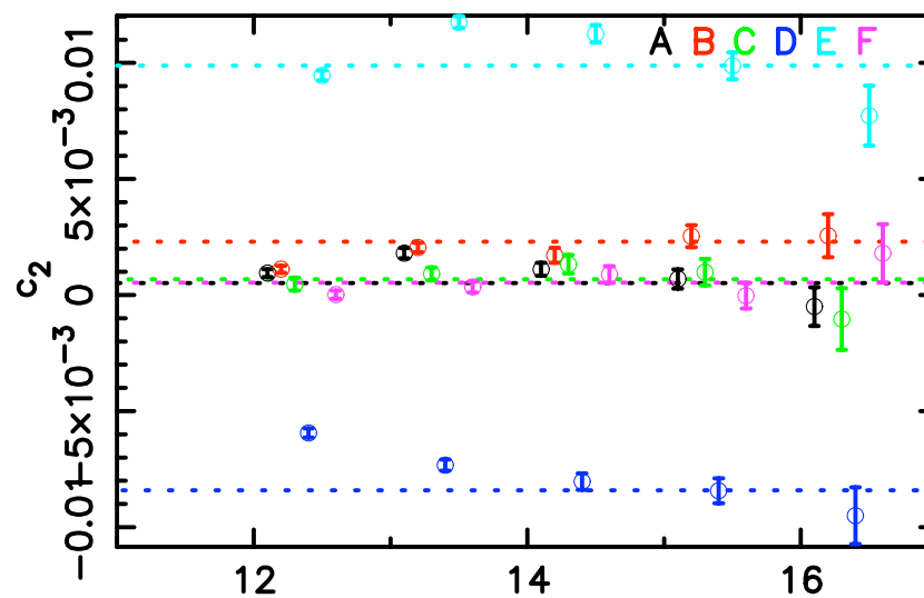
Magnitude
