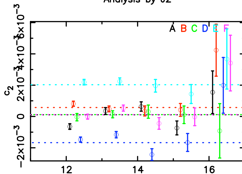
Magnitude
