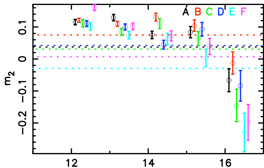
Magnitude
